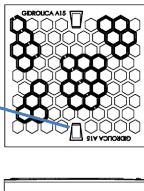
Решетка пластиковая «соты» A15
